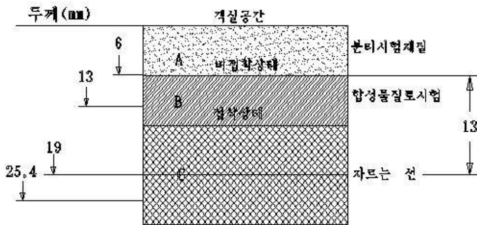
그 림 2 시편절단방법
