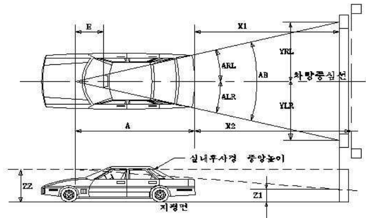
그림 7 실내후사경 시계범위
