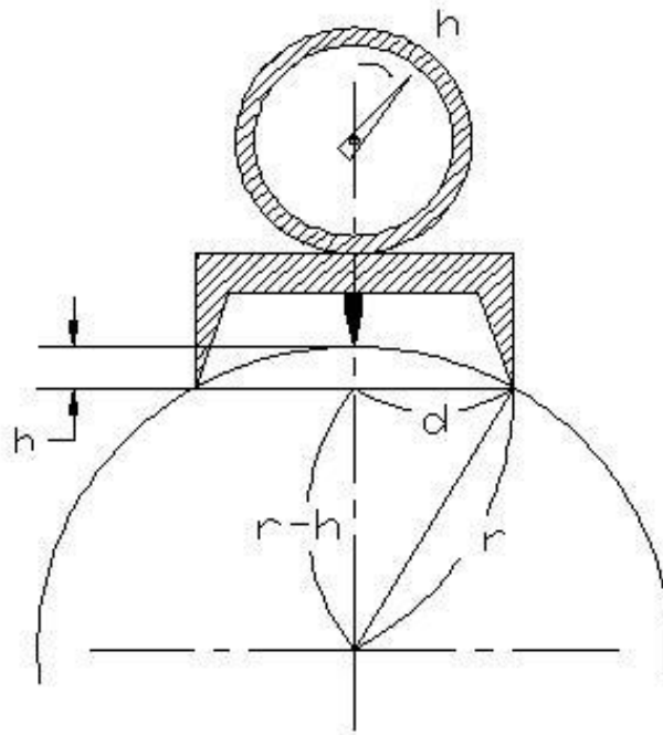
그림 10 곡률 반경 시험기
