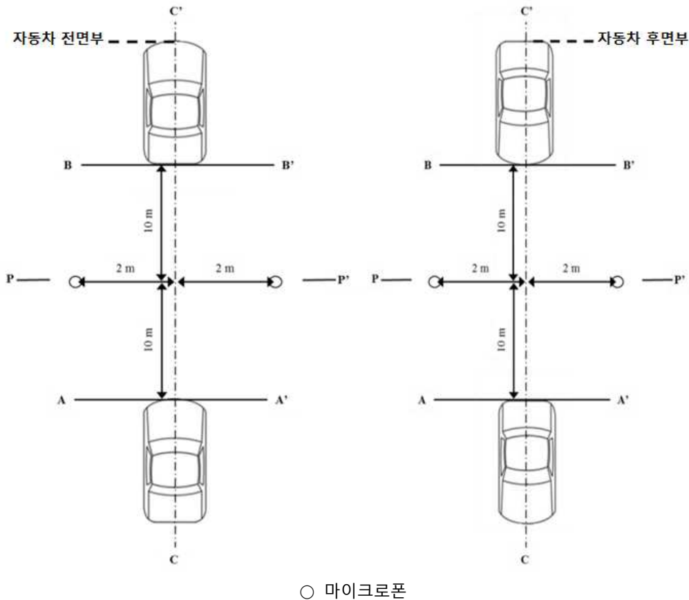
그림1a (전진주행)
