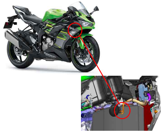
경음기 전기배선
