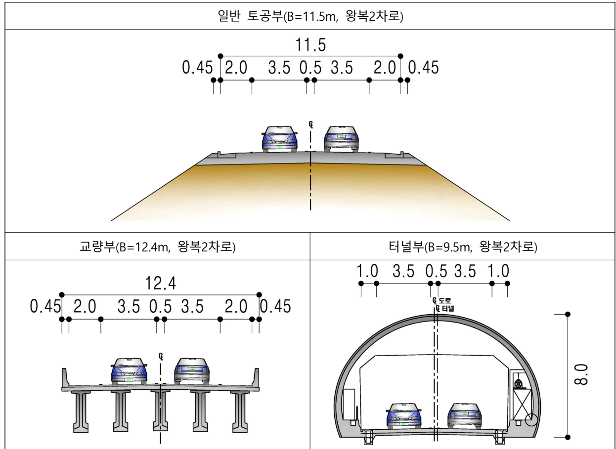
(그림 2.4-1) 표준 횡단면도
