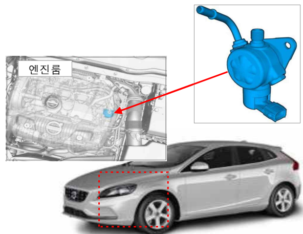
고압연료펌프
