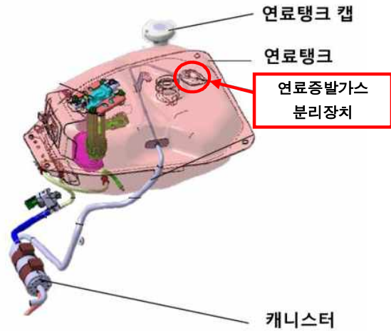
연료증발가스 분리장치
