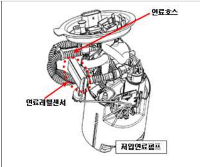
연료레벨센서
