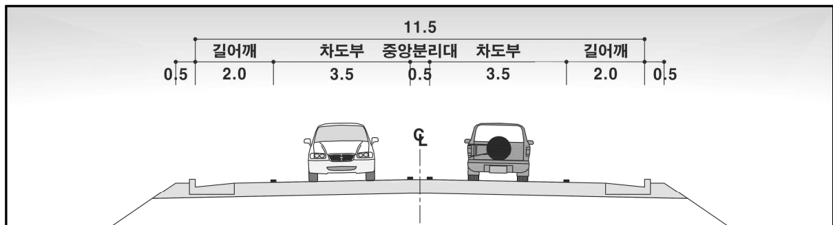
(그림 1.2-1) 도로표준횡단면도
