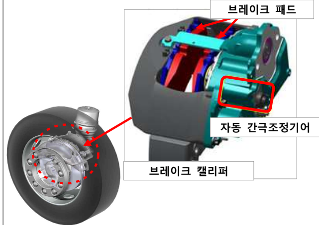
브레이크 캘리퍼 자동 간극조정기어
