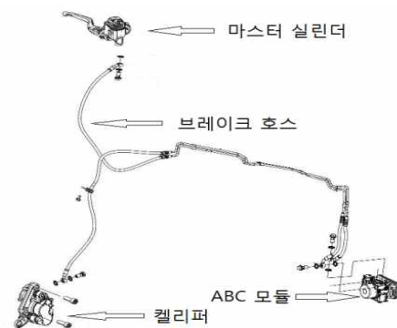
제동장치(브레이크 호스 및 마스터 실린더)
