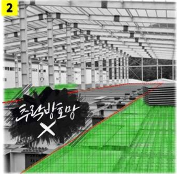
일부 구간 추락방호망 설치 X
