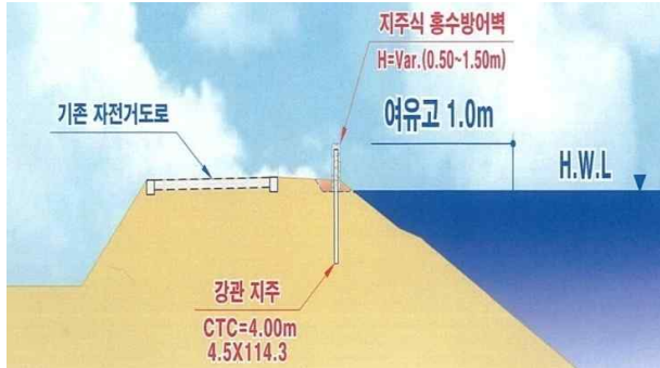
보축1지구(L=1.280km)
