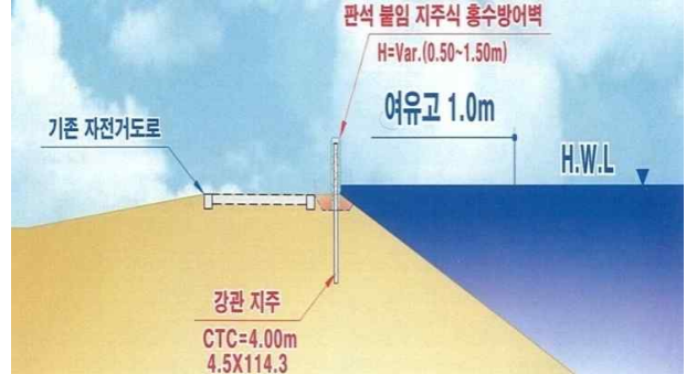
보축2지구(L=0.182km)
