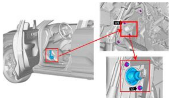
브레이크 제어장치
