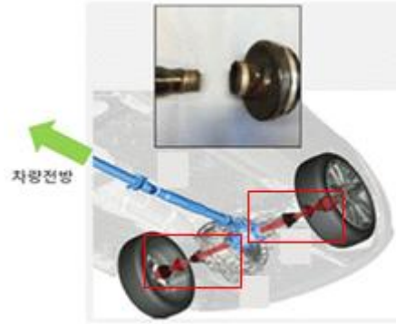
후륜 구동축(드라이브샤프트)
